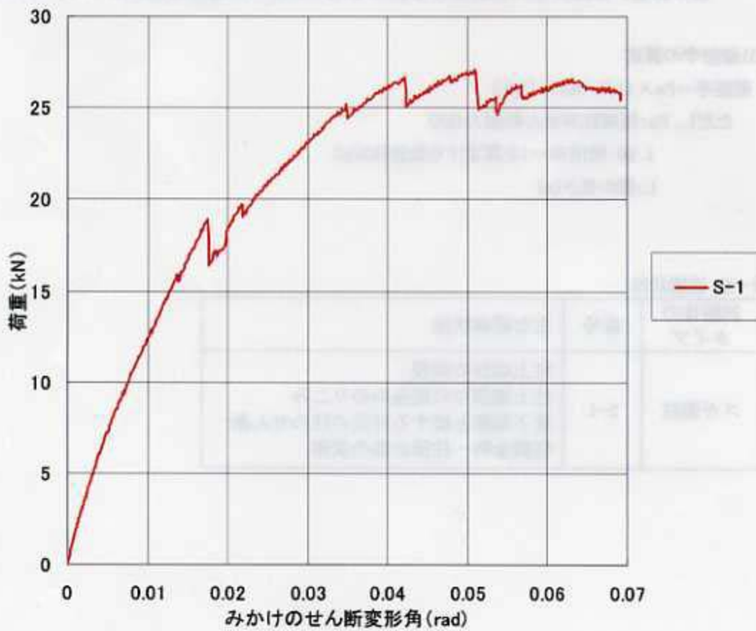
図-4 荷重-変形角包絡線
