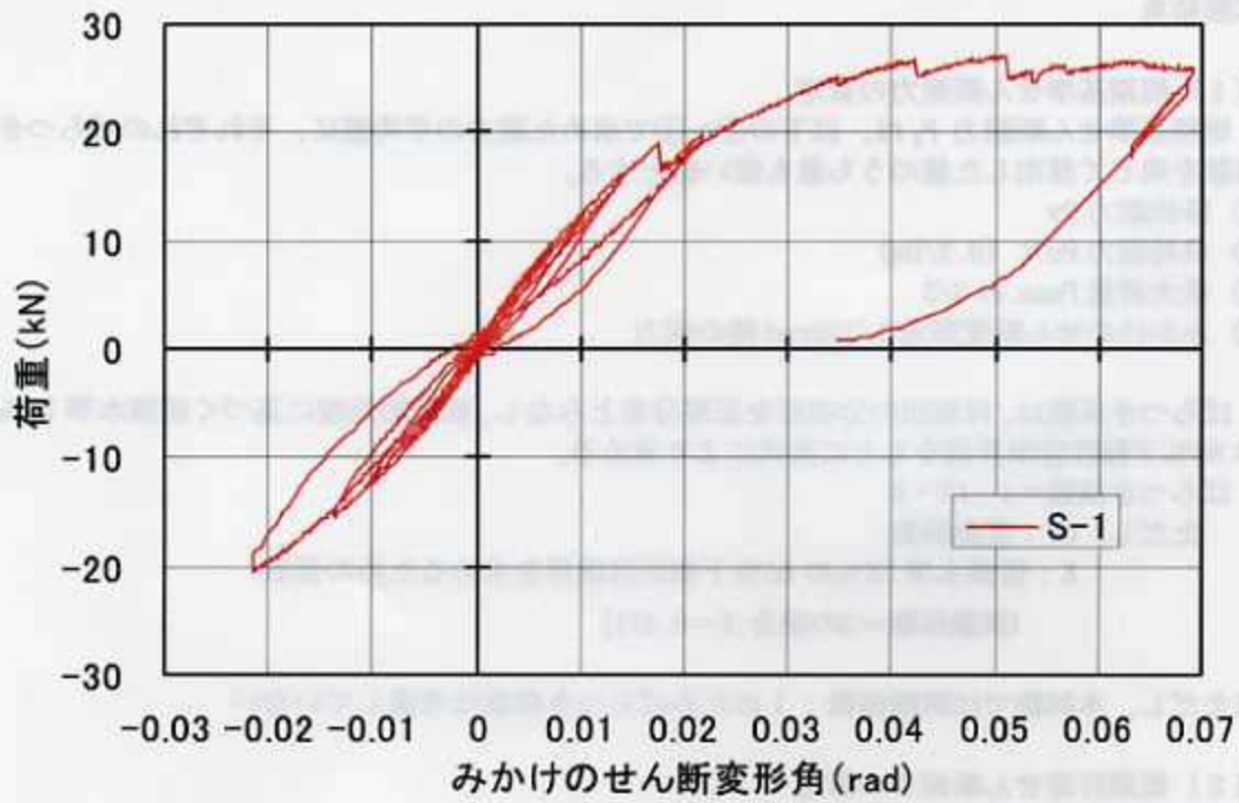
図-3 荷重-変形角曲線(S-1)
